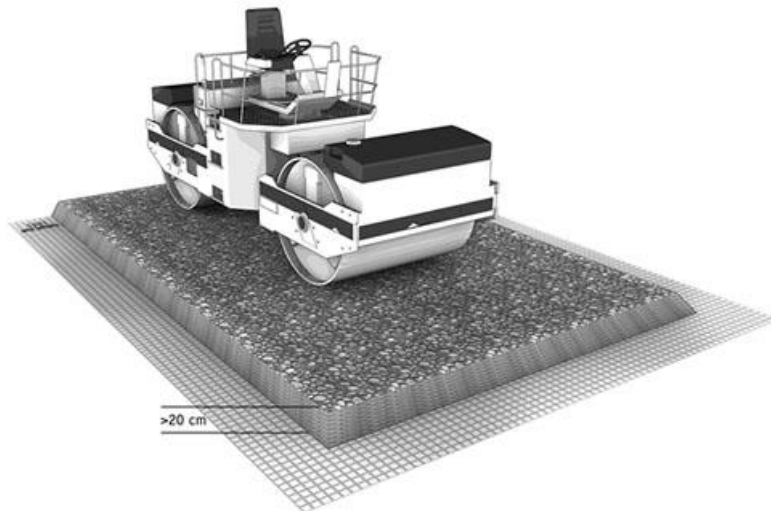
Zagęszczanie warstwy kruszywa na geokompozycie.
