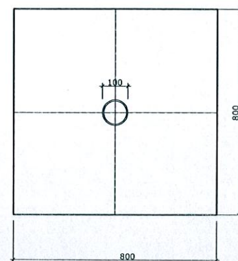
fundament słupa - rzut z góry
