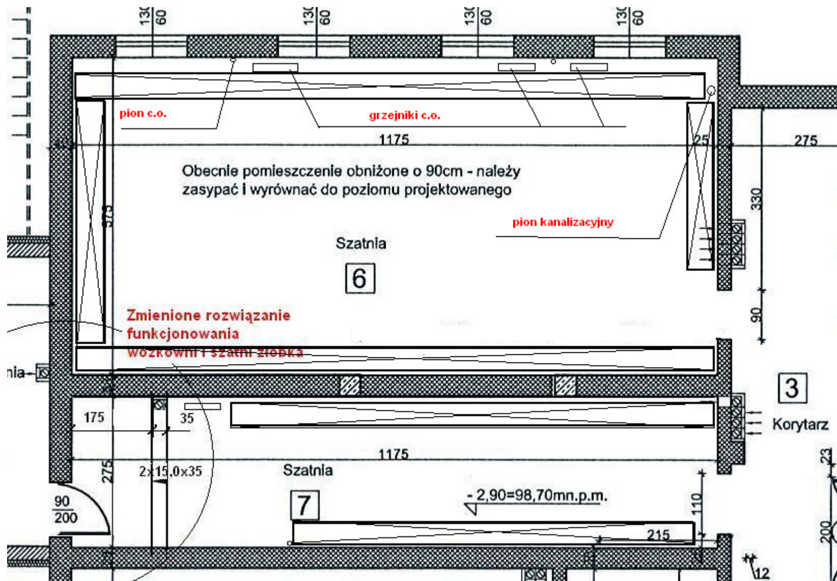
Szatnia nr 6 dla 120 dzieci i szatnia nr 7 dla 30 dzieci (proponowana zabudowa szatni) Przedszkole wraz z oddziałami żłobka w Lwówku
